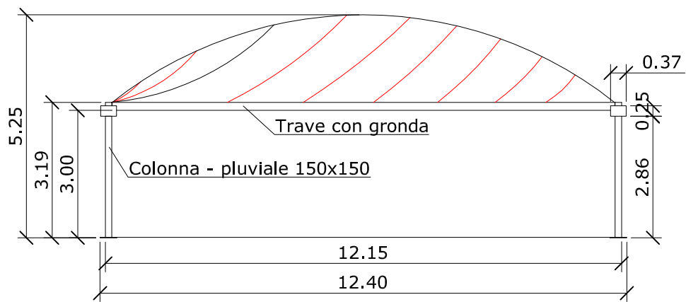
- PROSPETTO
